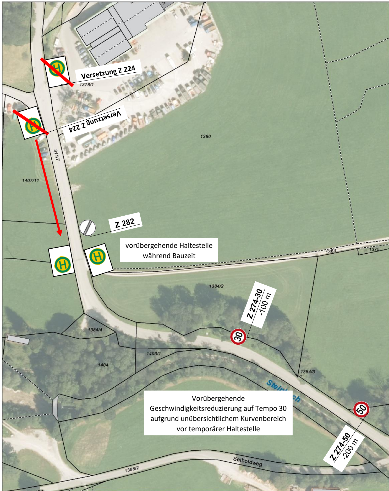
Lage-/Verkehrszeichenplan zu VAO 6301/2025-31
